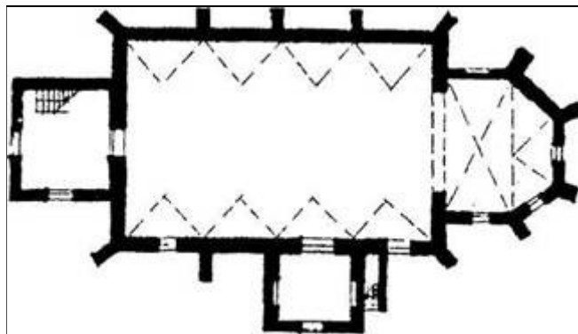
A szerencsi református templom alaprajza
